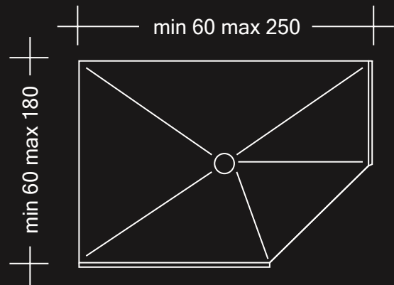
NICCHIA + SP
