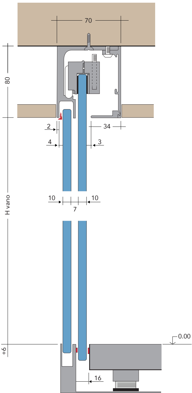
sezione A-X
