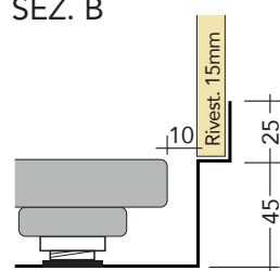
SEZ. B
