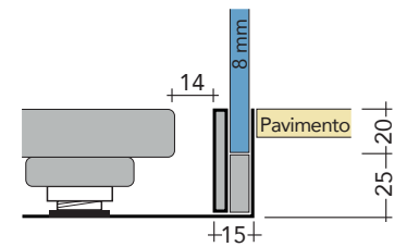
SEZ. E
