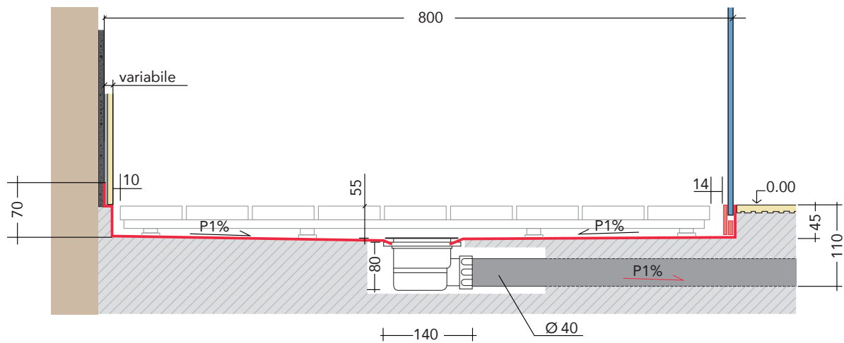
SEZIONE A-X
