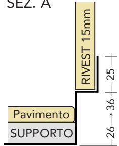
SEZ. A
