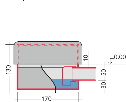
Prospetto "Scatola Sifonata"
