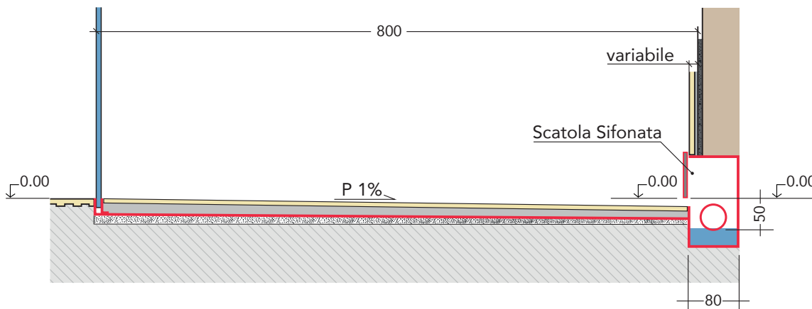
SEZ. A-X
