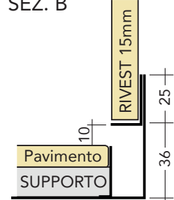
SEZ. B
