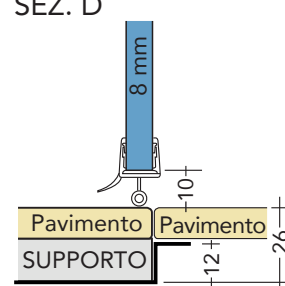
SEZ. D
