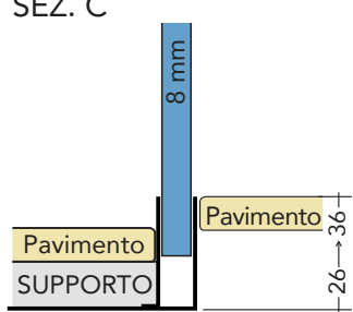
SEZ. C
