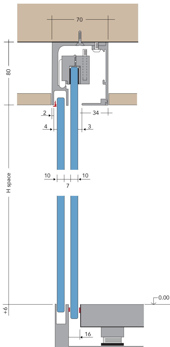
sezione A-X
